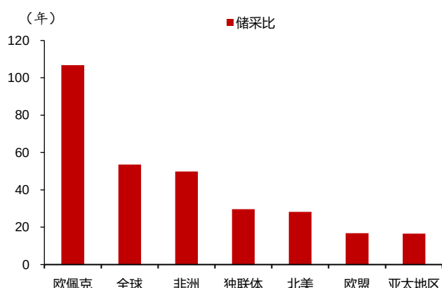
图6：全球原油储采比地区分布高度不均衡
